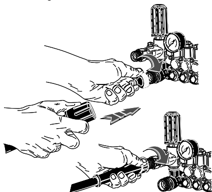
Wateraansluiting.
